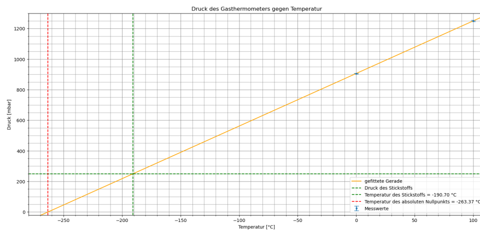
Abbildung 4.1: Druckwerte des Gasthermometers bei 0 °C und 100 °C.
